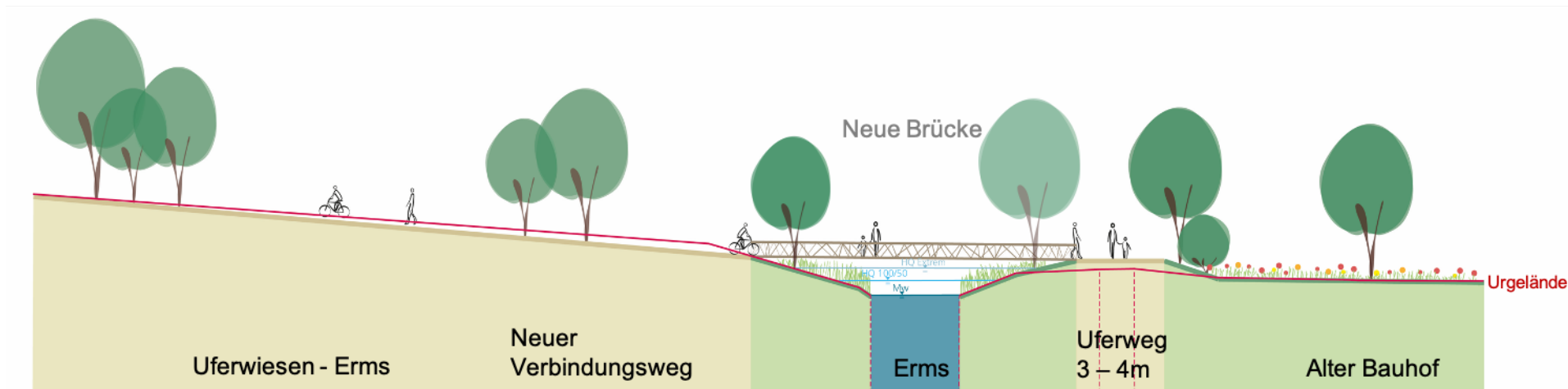
Schnitt 7 Ermswiesen – neue Brücke
